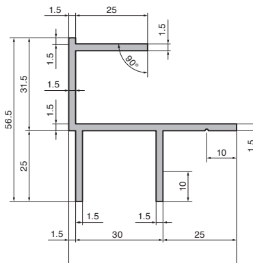
KP-30×1.5アルミFコーナー 図面
