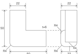
スポンジクッションコーナー
