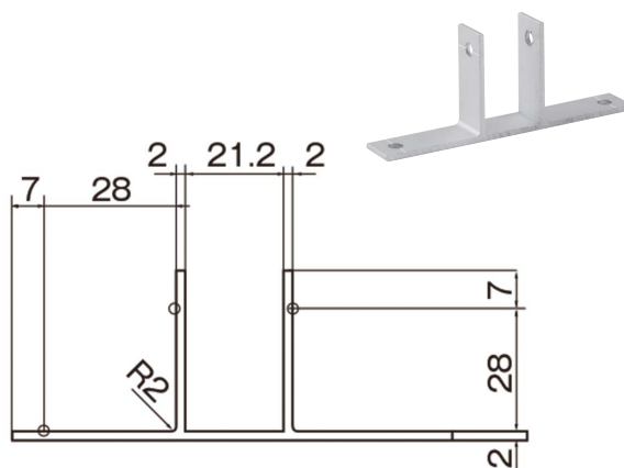
HE-20 用 T 型ブラケット
