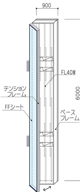
正面概要図
