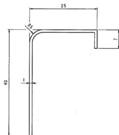
HE30、HE25兼用化粧カバー シルバー、ステンカラー、ホワイト、ブラック(艶消し)
