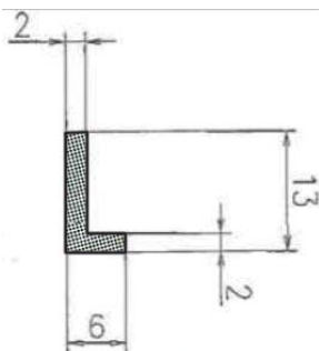
CU用アングル (2×6×13)
