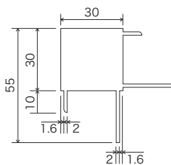
KP-30用L型コーナーブラケット
