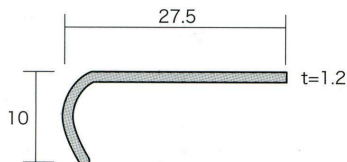
看板枠 35463
