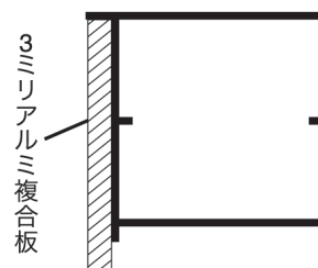
HE-27と3ミリ複合板かん合図
