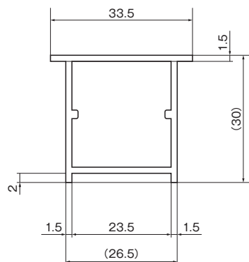
HE-27 用アルミコーナー、樹脂コーナー
