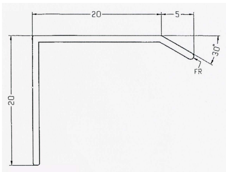
雨除けフレーム 225
