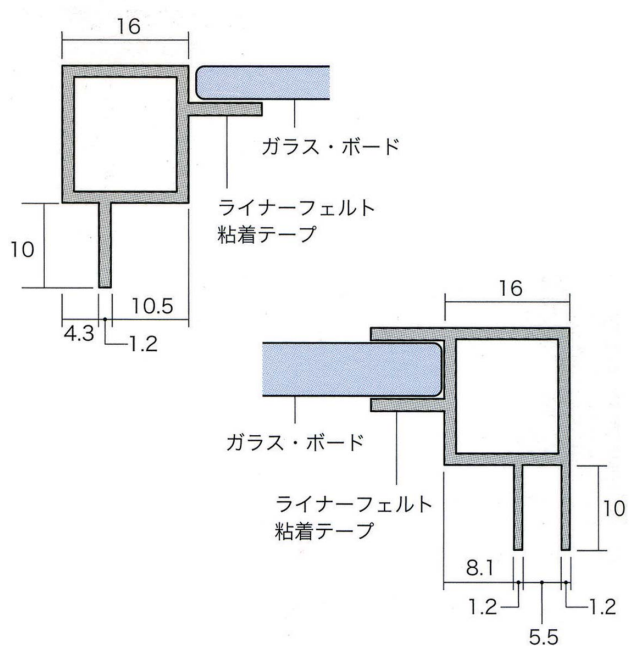
P/C システム 16
