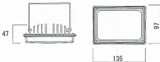
LED 投光器 エスポ 15W
