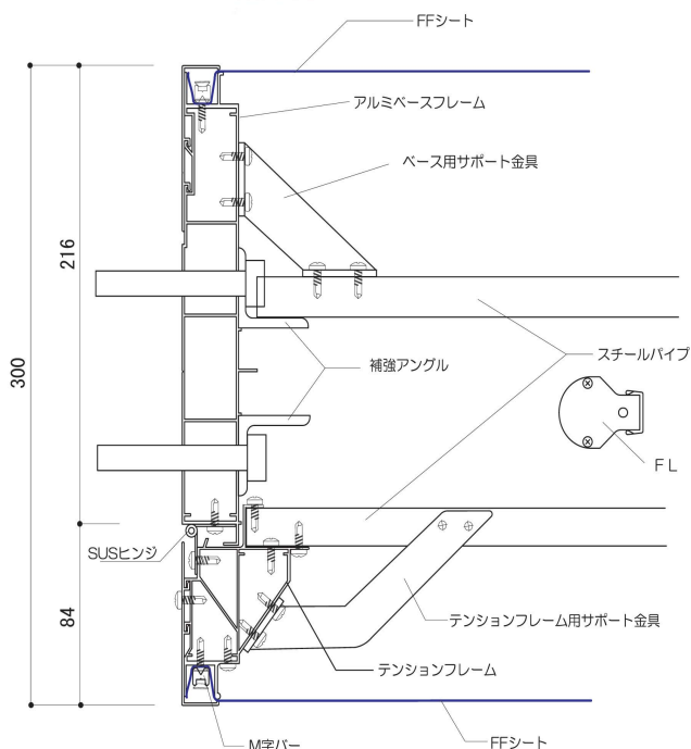
正面概要図
