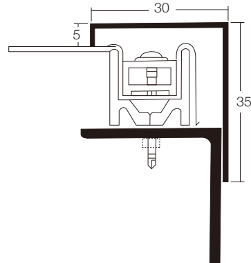
DS レールミニ + 看板枠 15755 かん合図
