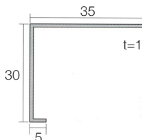
看板枠 15755 X 3640
