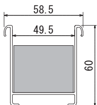
ポット 詳細図
