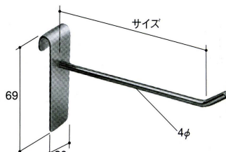
4φ ネットフック B型
