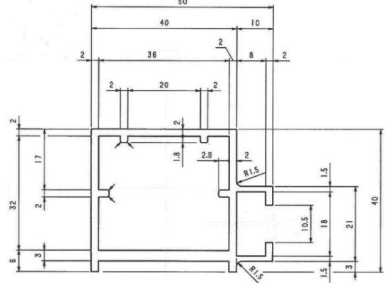
HE-40用中棧 B
