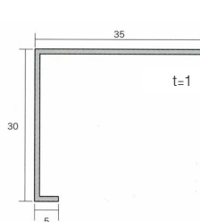
看板枠 15755
