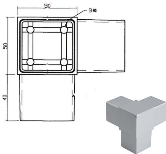
アルミダイキャスト三脚コーナー
