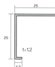
看板枠 15562
