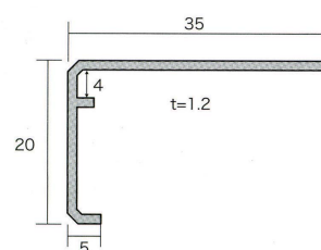
看板枠 3116 (25ミリ用)
