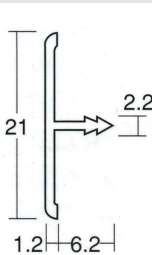
塩ビエッジ 21 白
