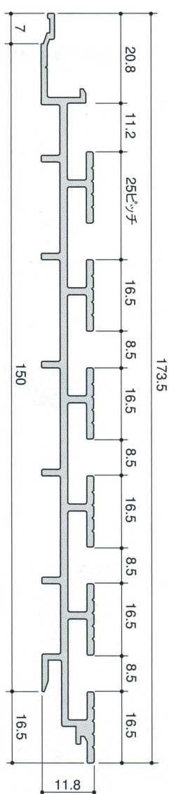
TFV下ホルダー
