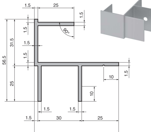
KP-30用L型コーナーブラケット
