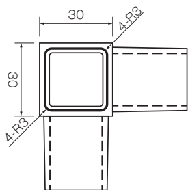
アルミダイキャスト三脚コーナー□2×30用
