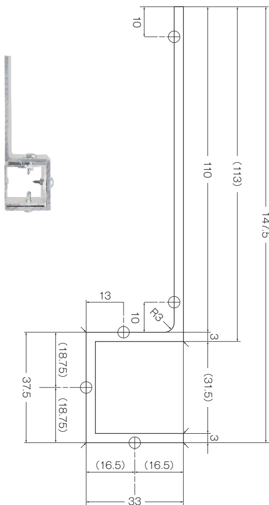
外照灯取付金具 野立用 断面図
