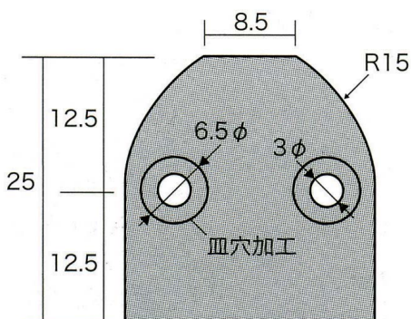
CU用フタ 上下1組
