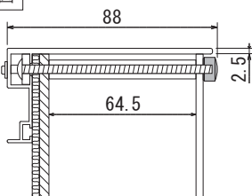
パネル 詳細図
