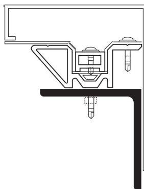
DS レール + 化粧カバーかん合図
