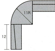
HM用コーナー
