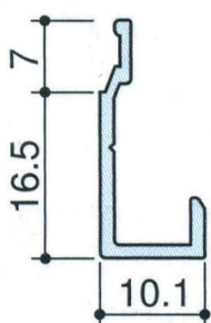
TFV下ホルダー
