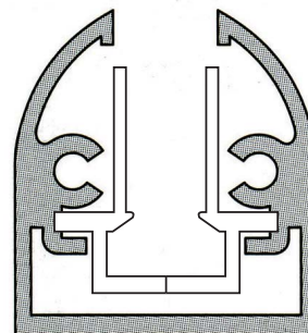
かんごう図
