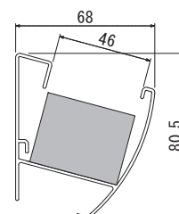
ポット詳細図 (GR4161、GR4162)
