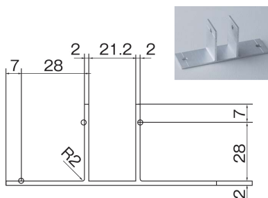
HE25用T型ブラケット
