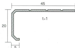
ボーダー 40角型
