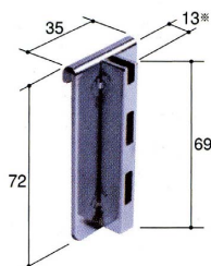
PH 棚柱 A
