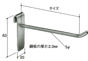
5φ ネットフック H型
