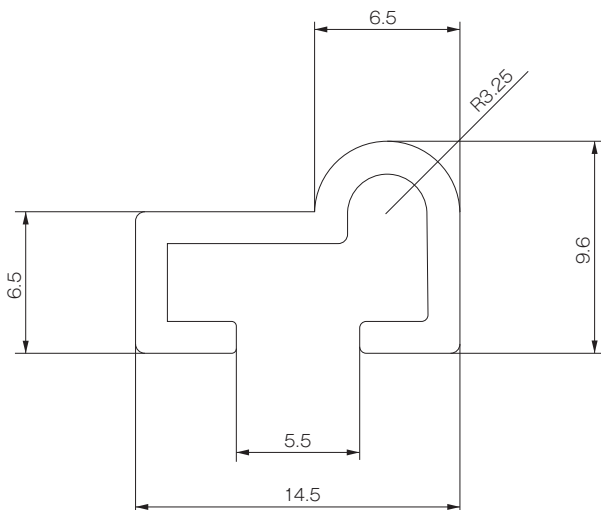
HFフレーム用吊り下げ金具 断面
