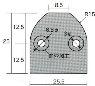
CU用フタ 上下1組
