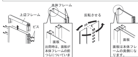
面板入れ替え簡単タイプへの組み替え方法
