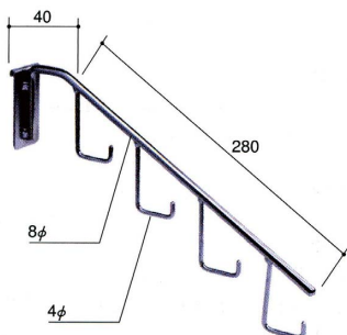
PH4 連バック掛
