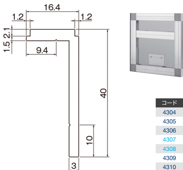
HE-20 用取付アングル
