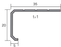
看板枠 35463
