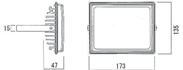
LED 投光器 エスポ 30W
