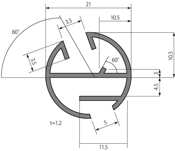
塩ビ 20 パイボトムバー
