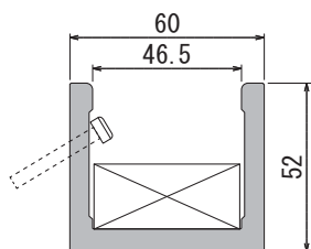
ポット詳細図
