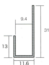
ステン 10 ミリ片長チャンネル X3M
