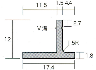
CUM、CU 兼用 Tバー
