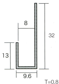
ステン 8 ミリ片長チャンネル X3M
