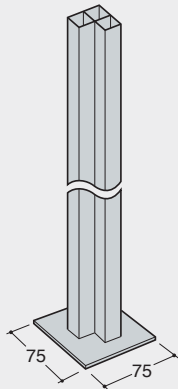
アーム AL-J4 L型 2,100mm
