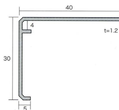
看板枠 39608
