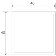
□2×40×40×4M シルバー
