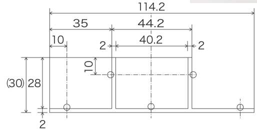
アルミダイキャスト三脚コーナー□2×40 用
