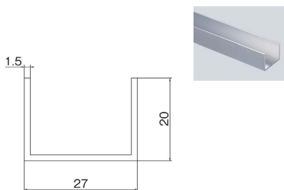
直ジョイント コ1.5X27X20X200
