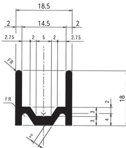
DS レール用化粧カバー
