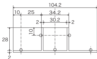
KP-30×1.5ミリ用アルミコーナー
