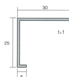
看板枠 15562
