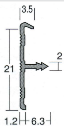
アルミエッジ A2-22.5
