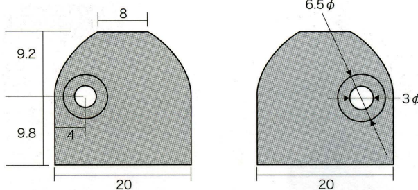
CUM用フタ 上下1組
