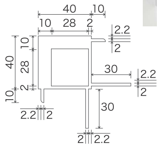
KP-40 用 L 型コーナーブラケット
