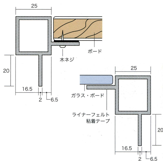
P/C システム 25
