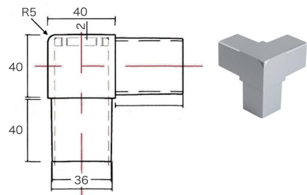
アルミダイキャスト三脚コーナー□2×40 用
