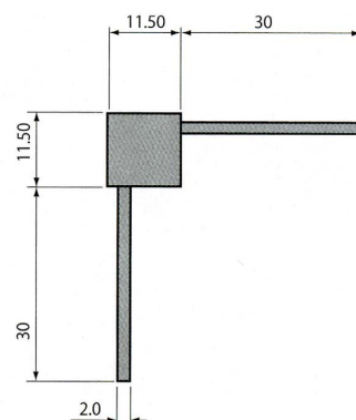
LED-70用コーナー (ポリカグレー色)
