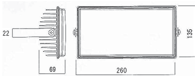
LED 投光器 エスポ 50W
