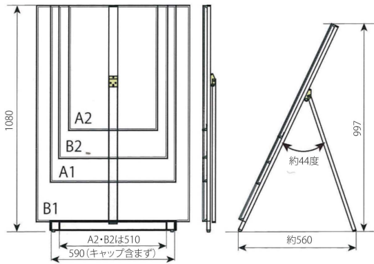
ロータイプ スリムエイト (シルバー)
