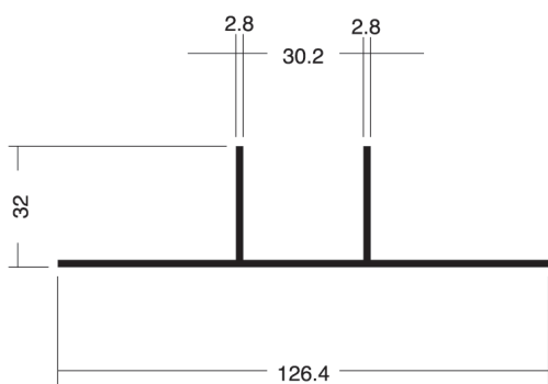
T 型ブラケット
