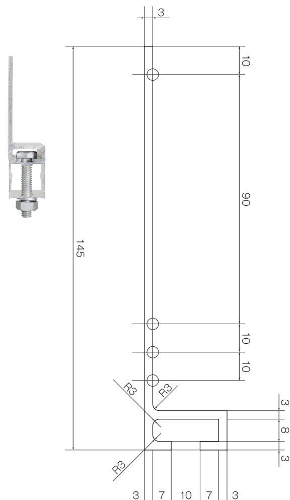
外照灯取付金具 壁付用 断面図
