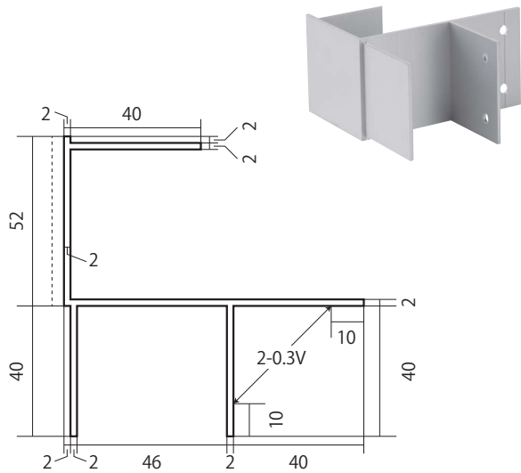
アルミダイキャスト三脚コーナー
