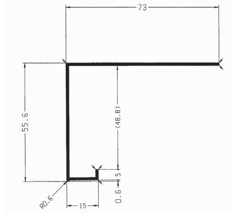
DS レールミニ + 看板枠 15755 かん合図
