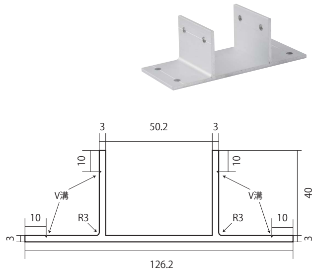
KP-50 用 T 型ブラケット
