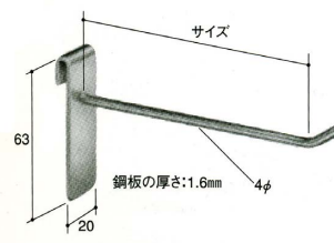
4φ ネットフック H型
