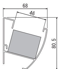
ポット 詳細図
