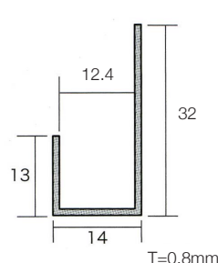
ステン 12 ミリ片長チャンネル X3M
