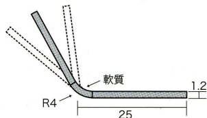
塩ビフリーアングル 25
