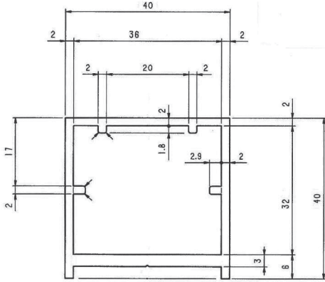
HE-40用中棧 A
