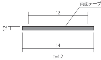
かんごう図
