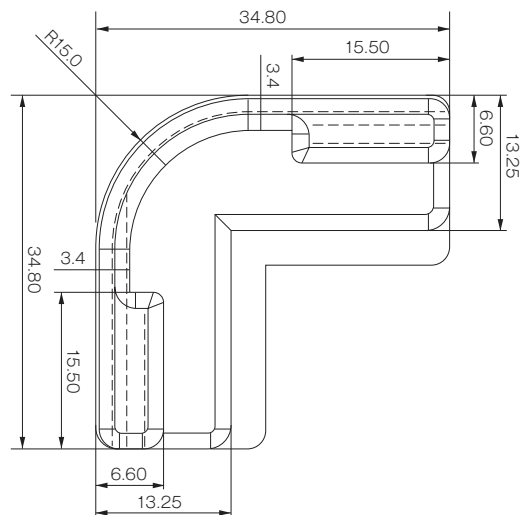
HFフレーム用キャップ
