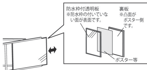
セット方法
